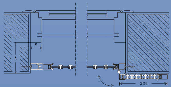
Κάτοψη: Τοποθέτηση πτυσσόμενου σε ρολό
