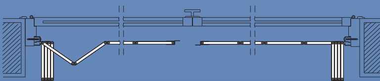
Κάτοψη: Εφαρμογή αντικατάστασης παλαιού παντζουριού
